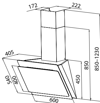
ODSÁVAČE PÁR
