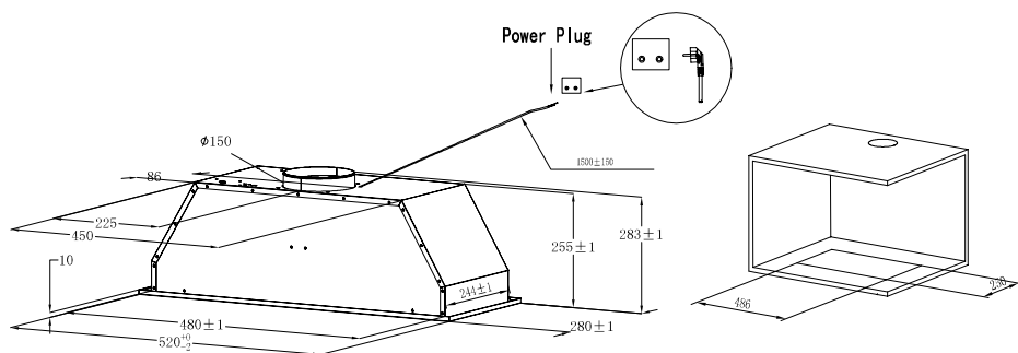
ODSÁVAČE PÁR
