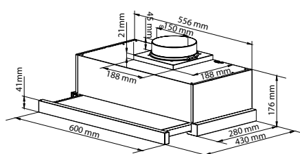
ODSÁVAČE PÁR
